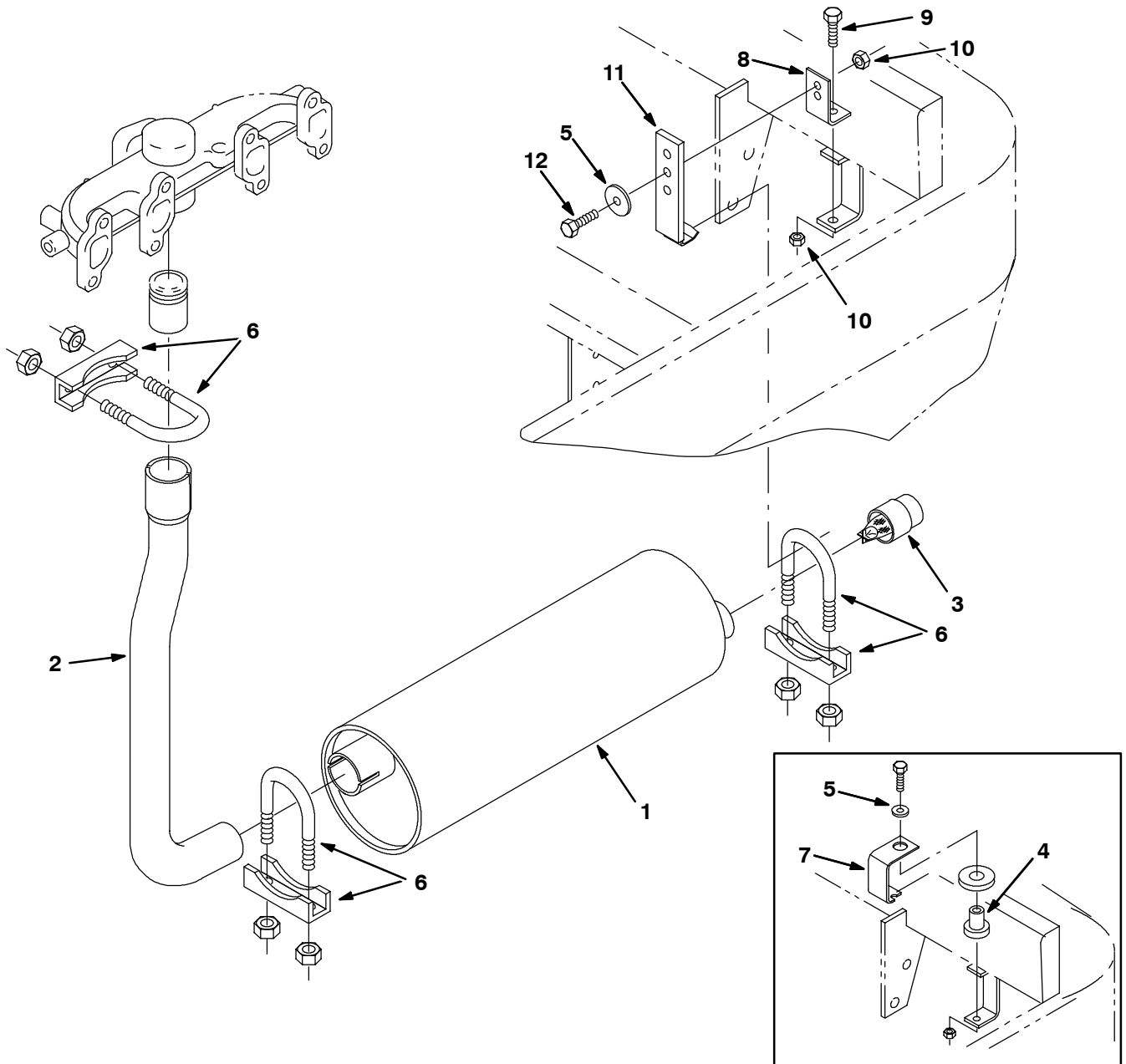
Fig. 24 - Muffler Group
