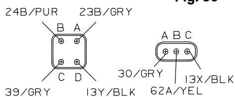
VIEW A-A
