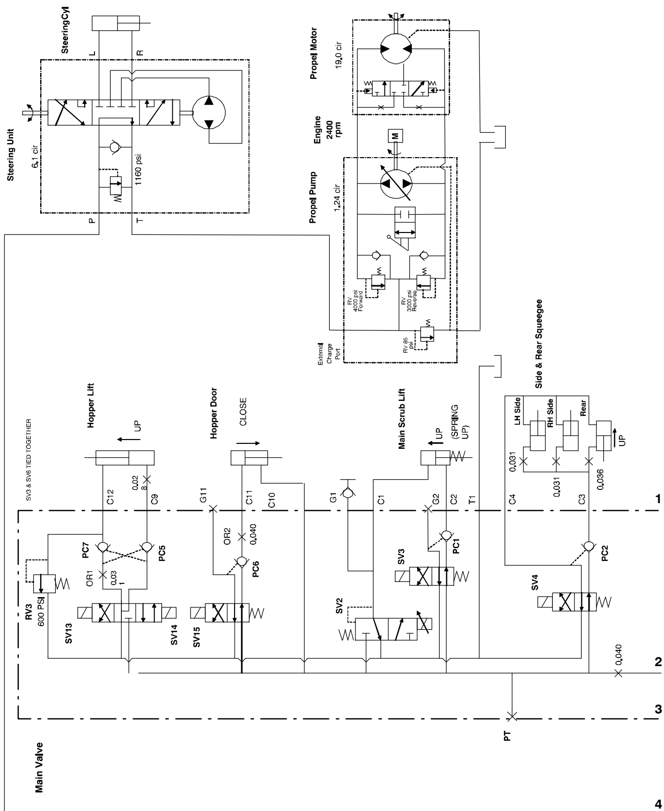
Fig. 62 - Hydraulic Schematic (002700-003297)
